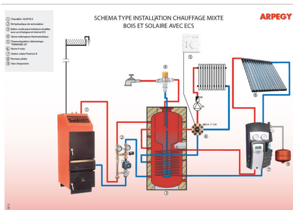
Shéma type installation chauffage mixte bois et solaire avec ECS
