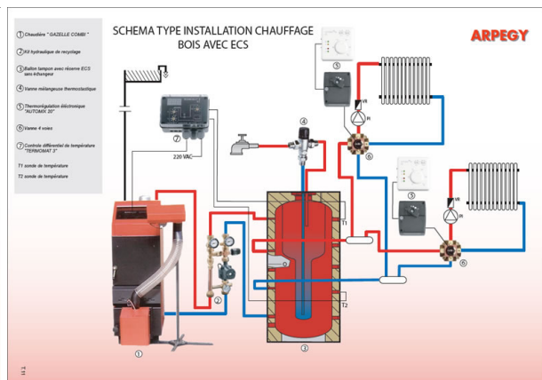
Schéma type installation chauffage bois avec ECS
